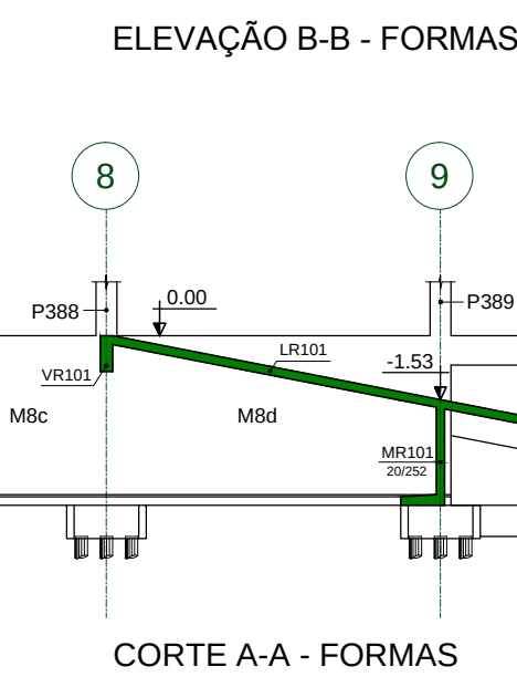
CORTE A-A - FORMAS
