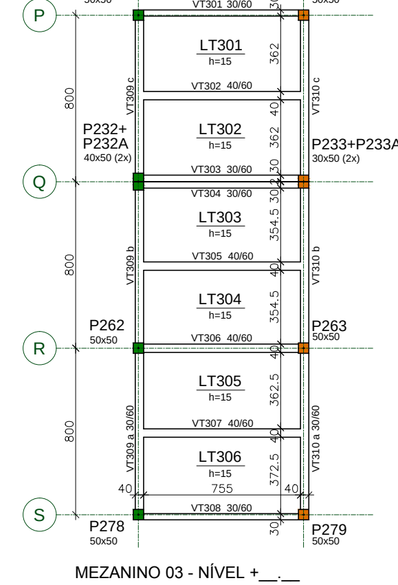
MEZANINO 03 - NIVEL +0.10
