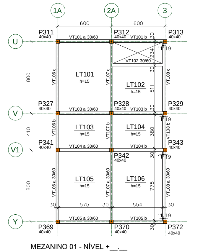
MEZANINO 01 - NIVEL +0.10
