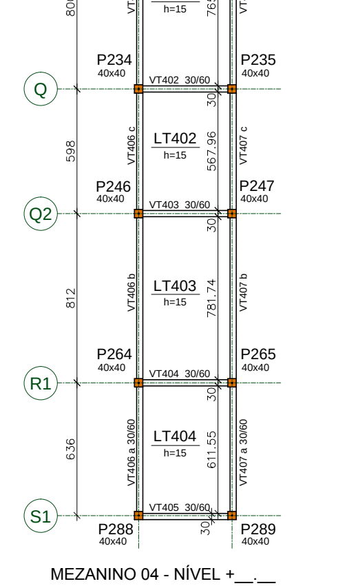
MEZANINO 04 - NIVEL +0.10
