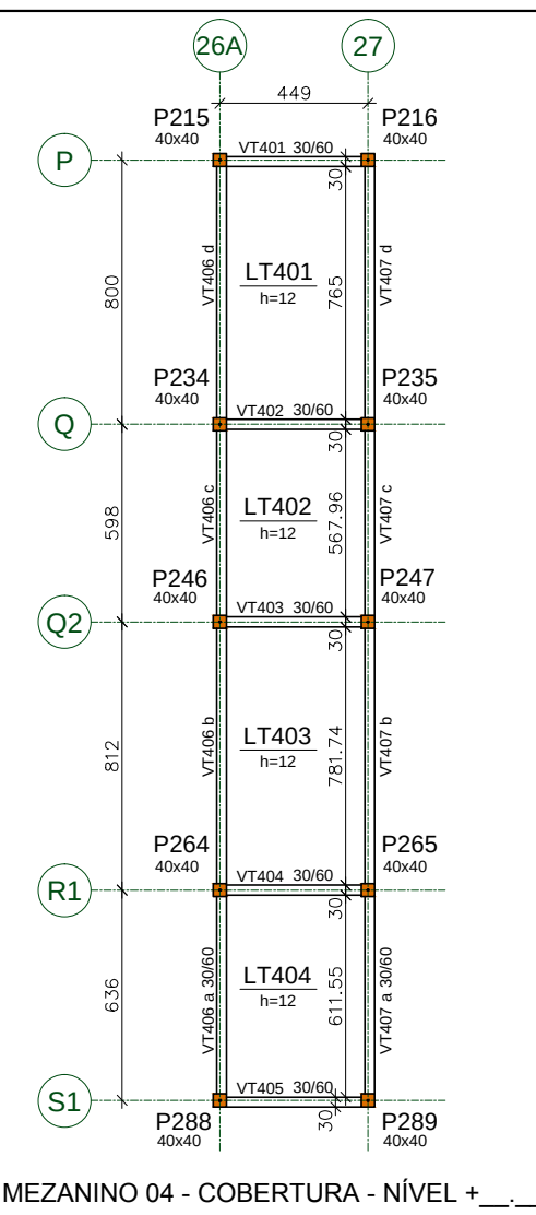
MEZANINO 04 - COBERTURA - NIVEL +0.10
