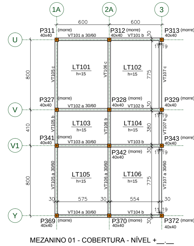
MEZANINO 01 - COBERTURA - NIVEL +0.10
