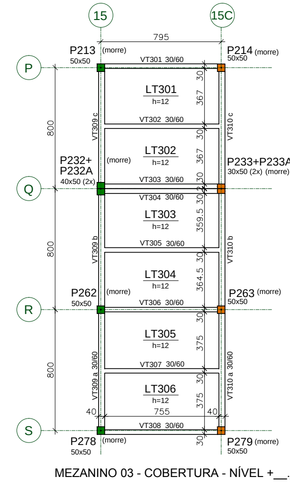
MEZANINO 03 - COBERTURA - NIVEL +0.10
