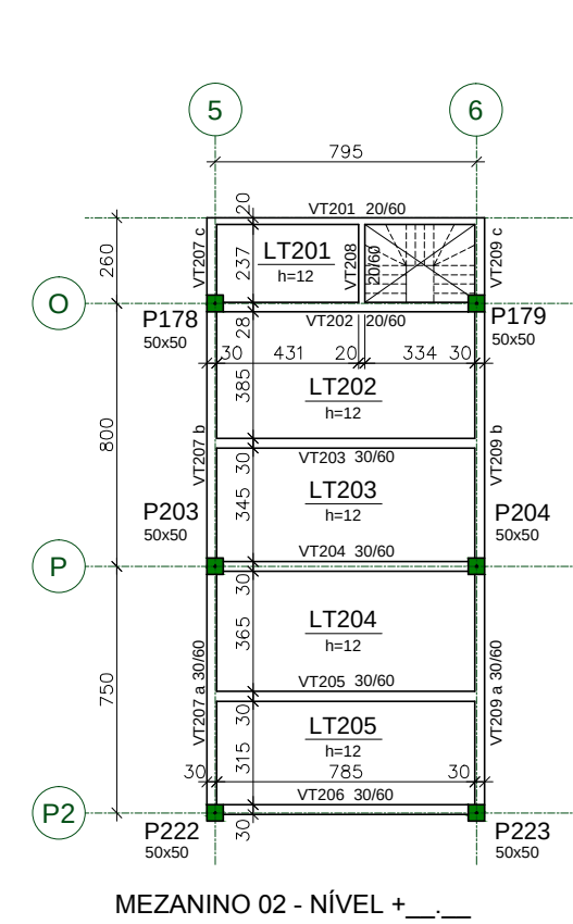
MEZANINO 02 - NIVEL +0.10
