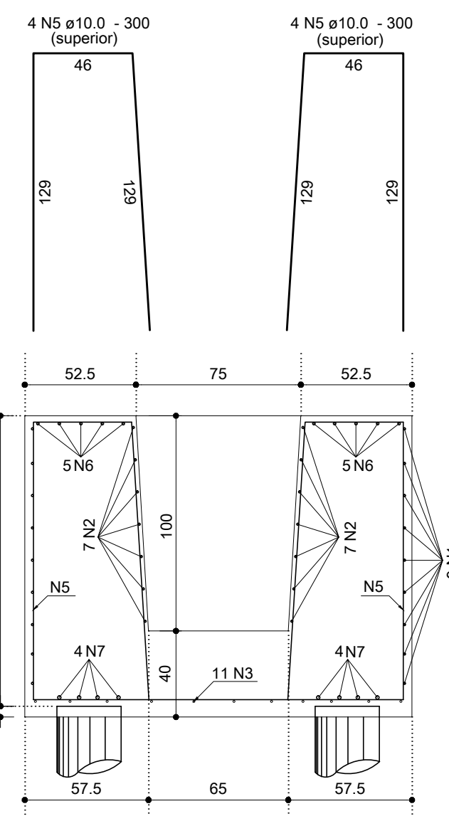
SEÇÃO B-B
